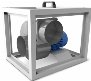
VENTILATEUR MOBILE ELECTRIQUE D 600 MM - 550 W - 9500 M3/H
